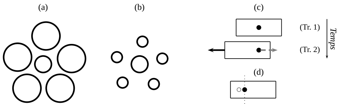
FIG. 2.1. – (Gauche) Illusion de Titchener . Le cercle central dans la configuration (a) est jugé plus petit que le cercle central de la configuration (b), alors que les deux ont en réalité le même diamètre. (Droite) Paradigme de mouvement induit et effet Roelofs . (c) Un cadre entourant symétriquement un disque positionné au centre de l'écran (Trame 1) est affiché peu de temps après dans une position légèrement décalée (Trame 2) par rapport au centre de l'écran, la position du disque n'ayant pas été modifiée. Le percept rapporté par les sujets est un déplacement du disque dans la direction opposée à celle du déplacement apparent du cadre (mouvement induit). Dans la configuration (d), le disque est situé dans la partie gauche d'un cadre décalé par rapport à l'axe sagittal du sujet, mais la position apparente du disque (modélisée ici par un cercle) semble être décalée dans le sens opposé à celui du cadre (effet Roelofs induit). Le segment vertical (en pointillés) représente l'axe sagittal du sujet.
