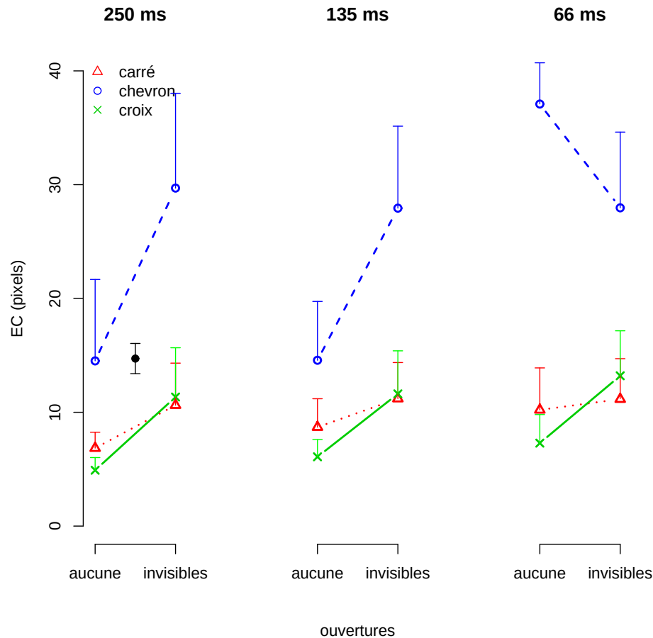
FIG. 4.13. – Erreur constante (+ 1 écart-type) représentée en fonction du type de forme(symboles) et de la visibilité des ouvertures, pour chacun des temps de présentation (de gauche à droite : 250, 133 et 67 ms). La valeur moyenne ( \pm l'erreur-type de l'interaction F_3 \times O_2 \times T_3 ) est représentée par le disque noir dans le graphique de gauche.
