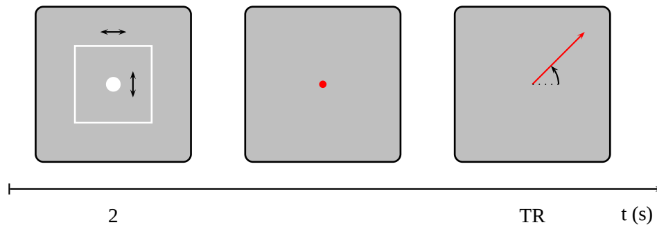
FIG. 5.2. – Illustration du déroulement d'un essai dans l'expérience 5a. On présente au sujet les deux stimuli en mouvement, la tâche consistant à évaluer la direction du mouvement du disque à la fin de l'essai, dès l'extinction des stimuli. Le sujet donne sa réponse en ajustant un vecteur rotatif.
