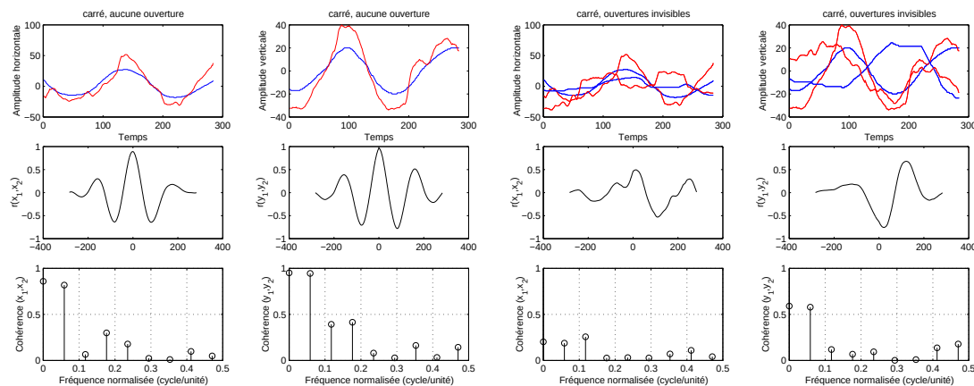
FIG. 3.13. – Corrélation croisée des trajectoires oculaires (en rouge) et manuelles (en bleu). La corrélation pour les deux composantes horizontales (gauche) et verticales (droite) indiquée est indiquée dans les graphiques du milieu, dans le cas du carré pleinement visible et masqué par des ouvertures invisibles. Les coefficients de corrélation estimés sont normalisés. La fonction de cohérence estimée pour les fréquences normalisées est indiquée dans le diagramme du bas.
