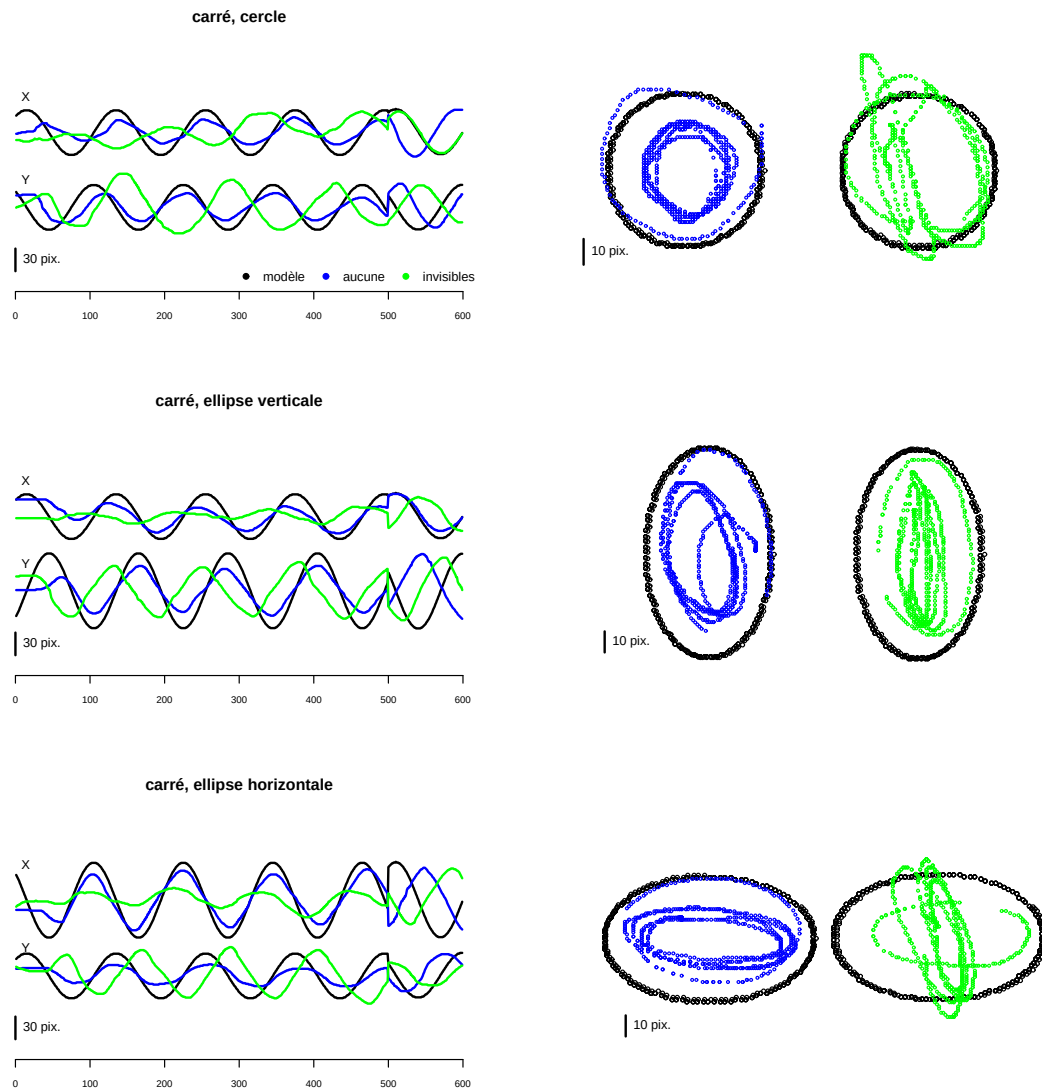
FIG. 3.8. – Exemples de trajectoires réalisées par un même sujet dans les tâches de poursuite avec les trajectoires imposées cercle (haut), ellipse verticale (milieu) et ellipse horizontale (bas), dans les conditions aucune ouverture (en bleu) et ouvertures invisibles (en vert). La trajectoire de la cible est indiquée en noir. Le décours temporel des composantes horizontales et verticales est indiqué dans le panneau de gauche, tandis que les trajectoires 2D sont reportées sur le panneau de droite.
