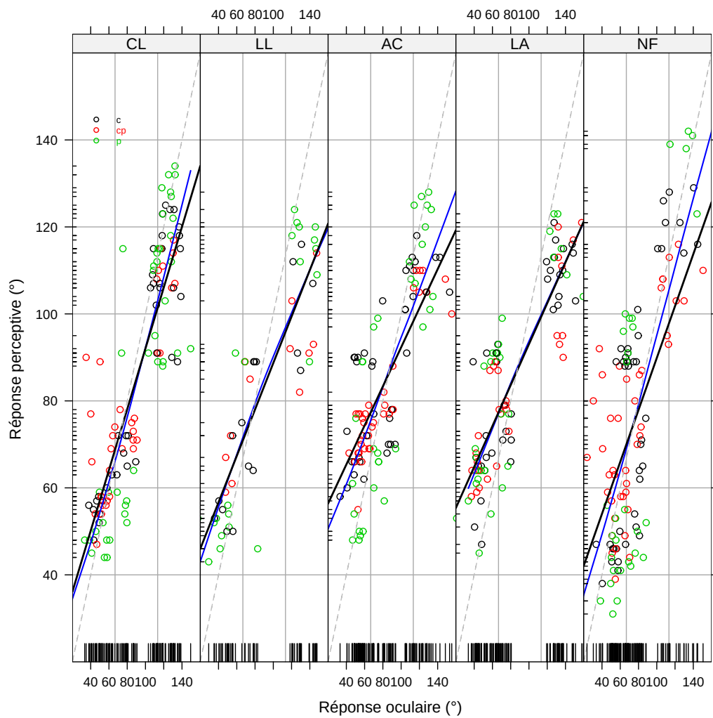
FIG. 6.7. – Distribution bivariable des réponses perceptives et oculaires ( n = 5 ) en fonction du type de stimulus ( c , noir, c+p , rouge, p , vert). La droite en pointillés gris indique la droite de pente unité. Les droites de couleur bleue et noire représentent des droites de régression pondérée et ordinaire, respectivement.
